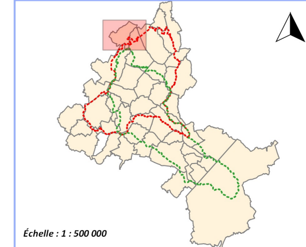
Carte d'aléa des phénomènes de ruissellement et de débordement dans la vallée de la Rhonelle et de ses affluents
