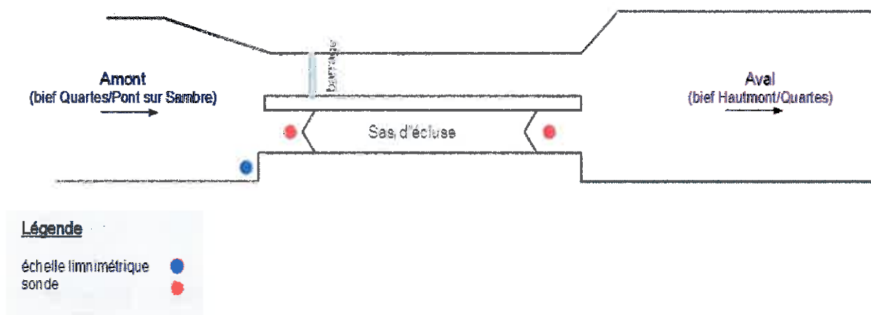
Fig.17 : Positionnement de l'instrumentation à Quartes
