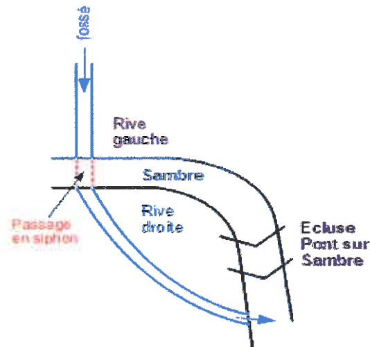
Fig.10 :Schéma du passage en siphon sous la Sambre canalisée
