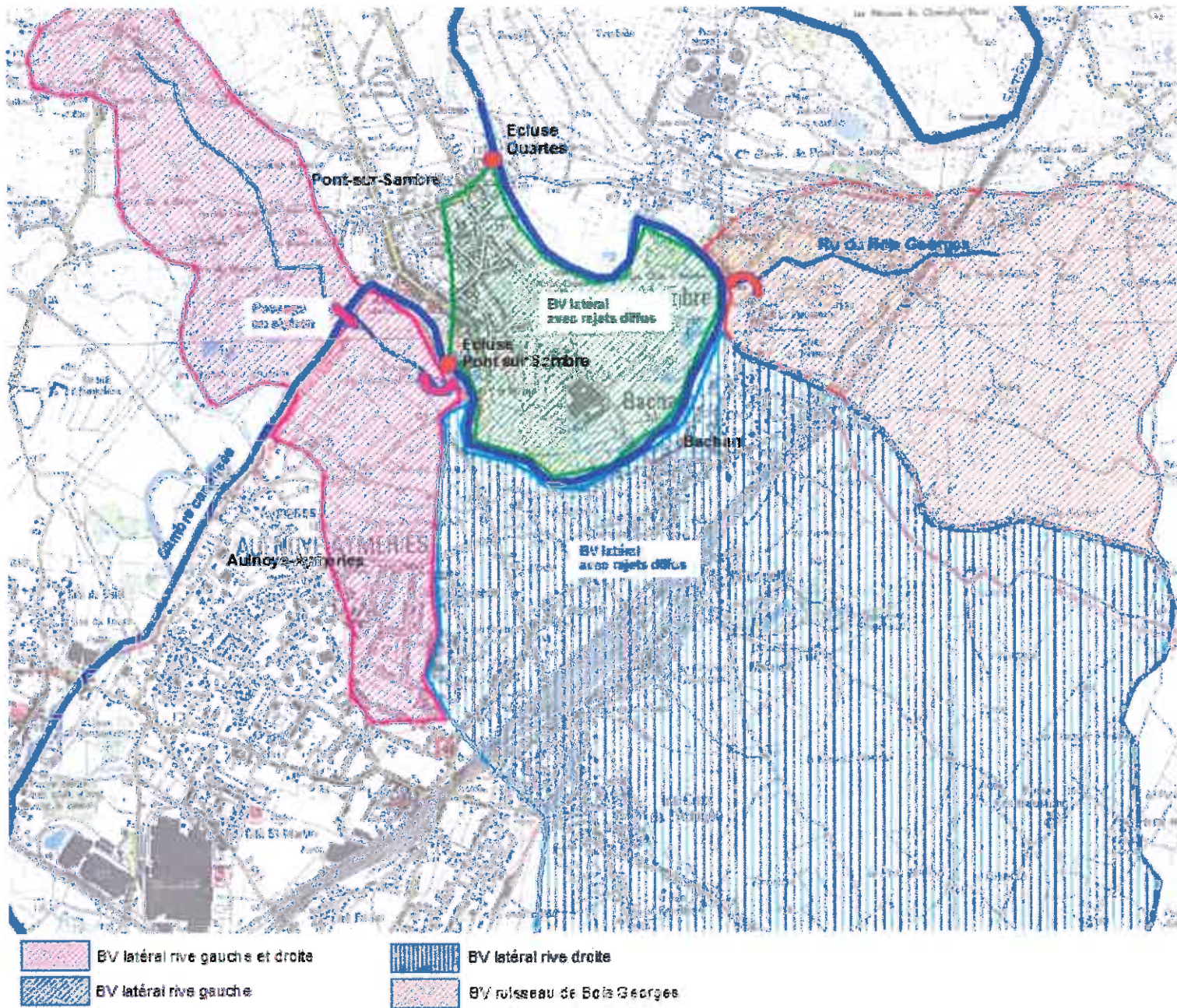
Fig.7 : Bassins versants rive gauche/rive droite de la Sambre canalisée sur le bief Quartes/Pont-sur-Sambre
