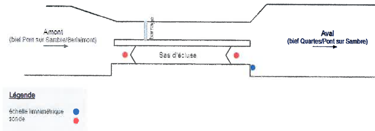
Fig.16 : Positionnement de l'instrumentation à Pont-sur-Sambre
