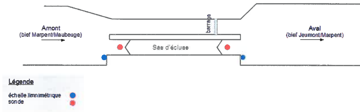
Fig.18 : Positionnement de l'instrumentation à Marpent
