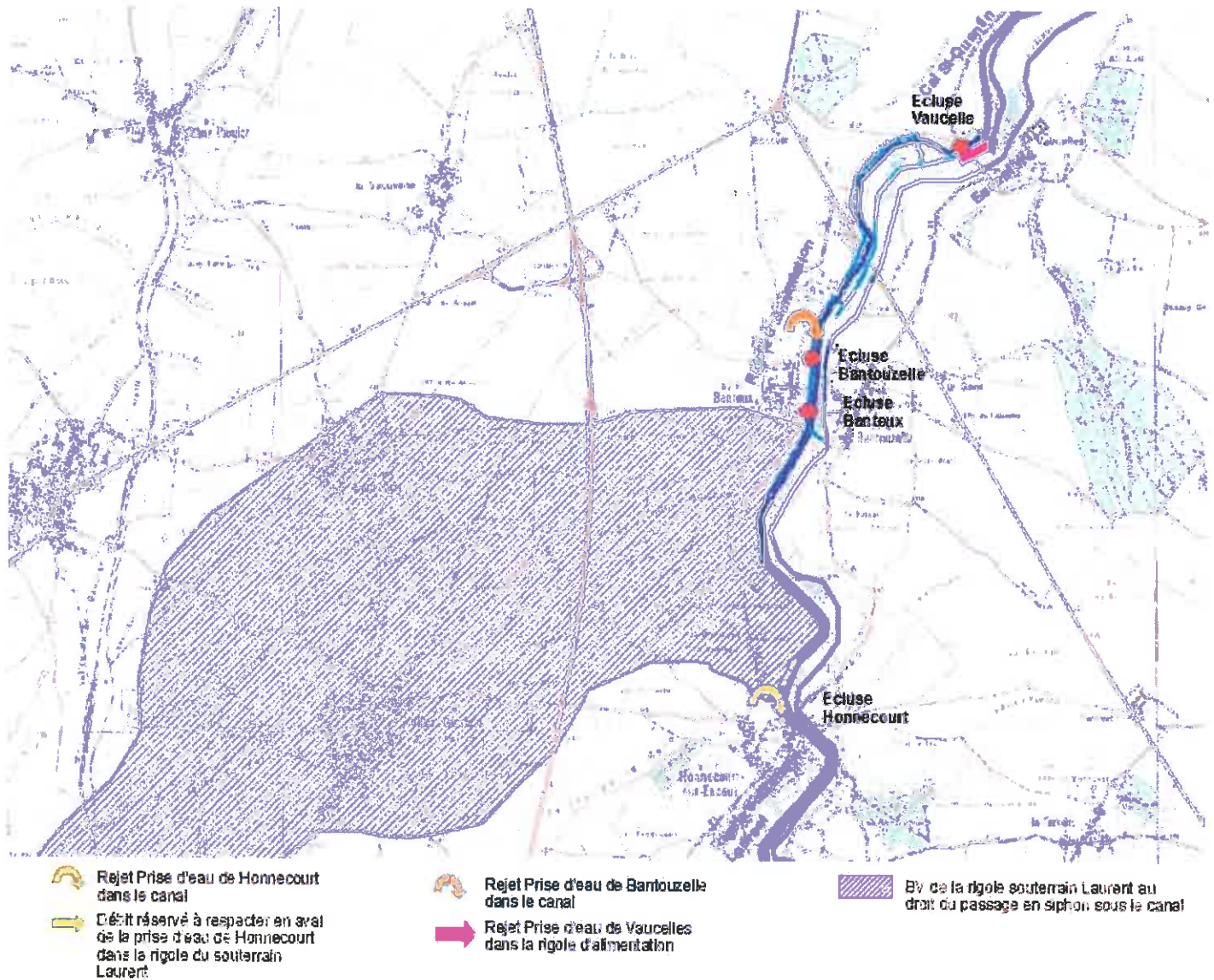
Fig.25 : Bassin versant en amont du passage en siphon de la rigole du souterrain Laurent
