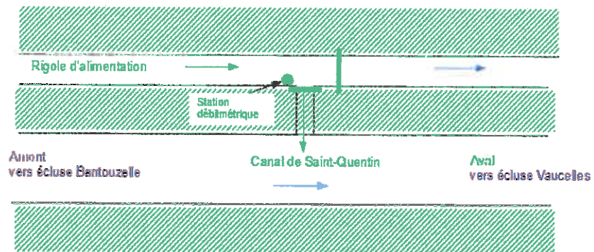
Fig.22 : Positionnement de la station débitmétrique
