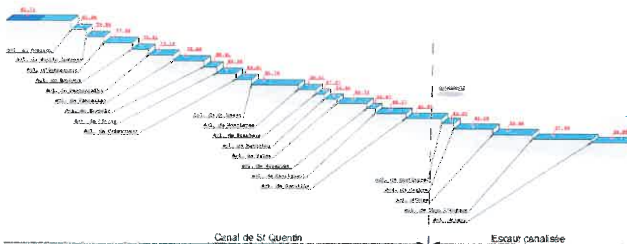
Fig. 4 : Profil en long du Canal de Saint-Quantin (extrait du schéma hydraulique de VNF Nord-Pas de Calais)
