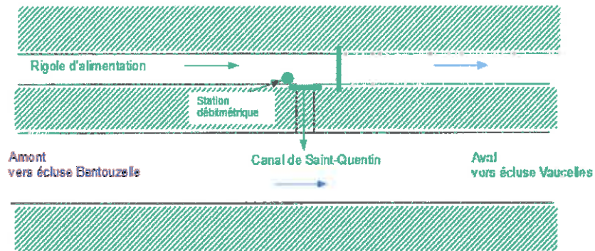
Fig.22 : Positionnement de la station débitmétrique
