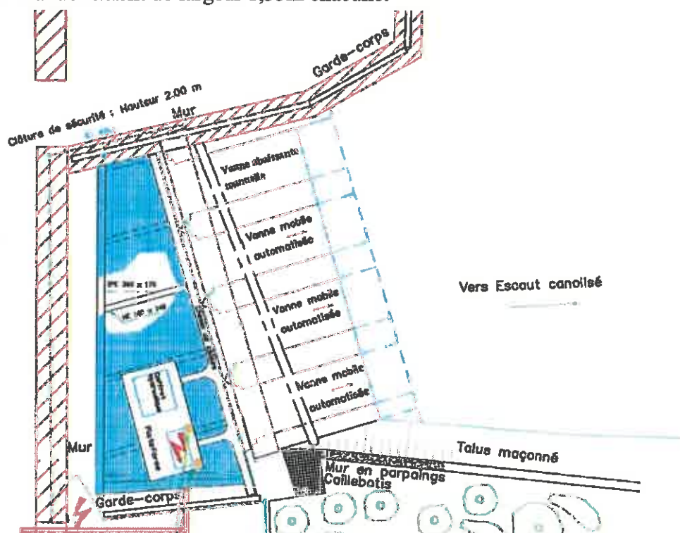
Fig.10 : plan du barrage
