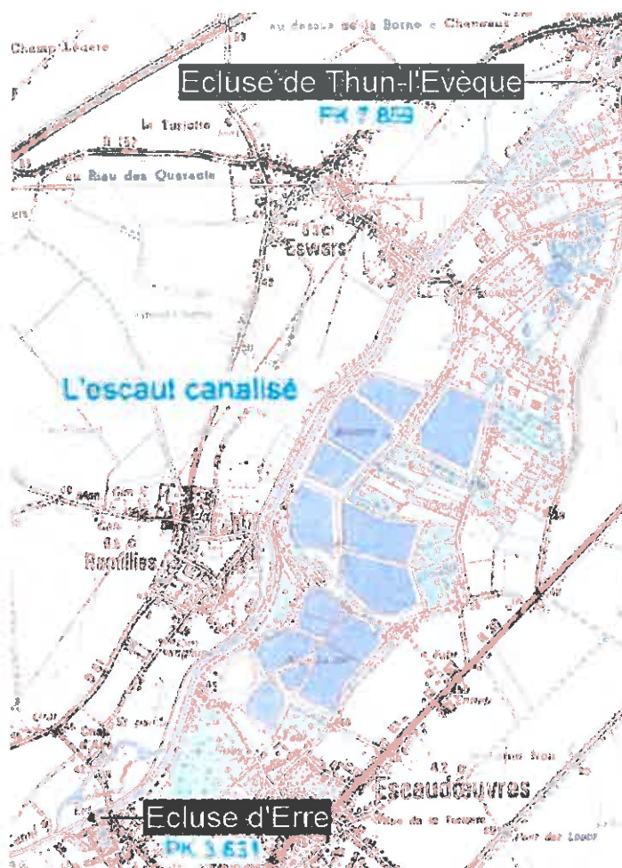
Fig.7 : Présentation du bief Erre/Thun l'Évêque
