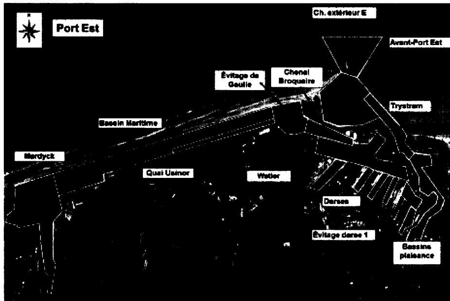
Localisation des zones de dragage sur le Port Est de Dunkerque
